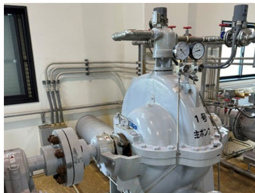
Fig. 1 上流端の揚水機場の様子
